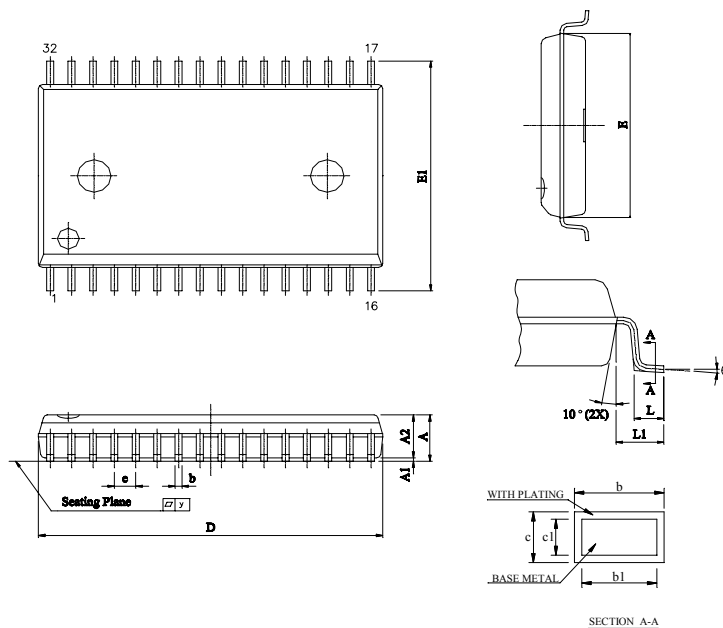
SOP -32
