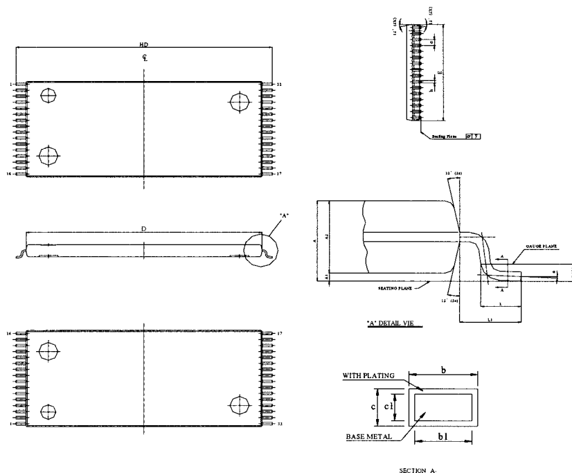
TSOP - 32
