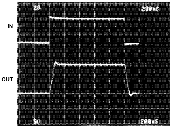
Horizontal Scale: 200ns/Div. Vertical Scale: 2V/Div. Input, 5V/Div. Output
