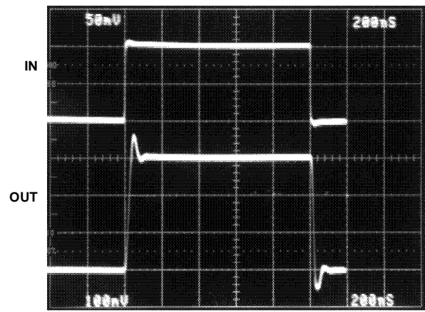
Horizontal Scale: 200ns/Div. Vertical Scale: 50mV/Div. Input, 100mV/Div. Output
