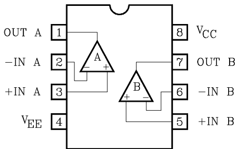
KIA4558P, KIA4558F
