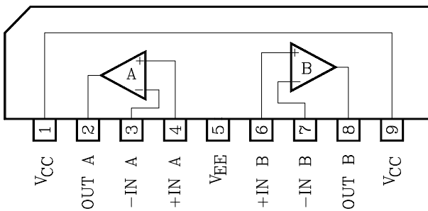
KIA4558S
