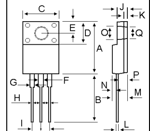
ITO-220
