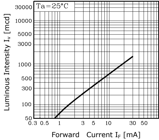
Fig. 2 I_V - I_F
