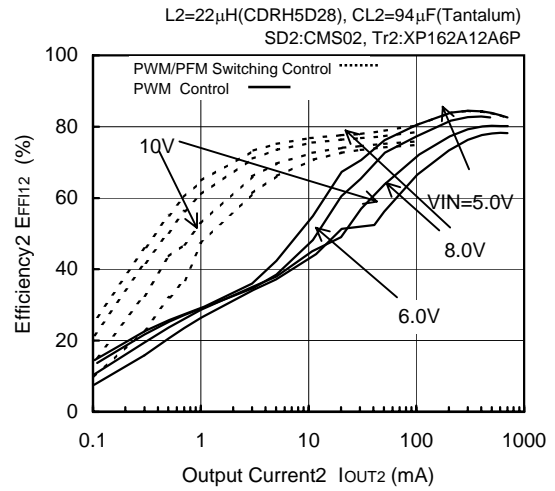
FOSC=300kHz, VOUT2=2.5V
