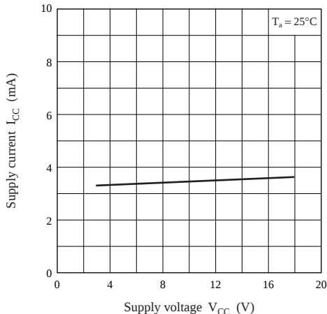
I_{CC} - V_{CC}
