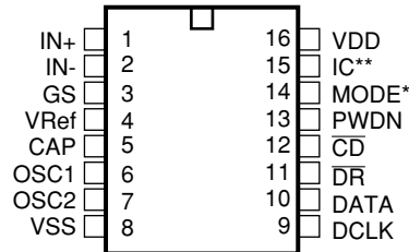
16 PIN SOIC
