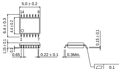
BU4066BCFV
