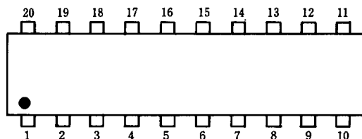
NJM2366G NJM2366V
