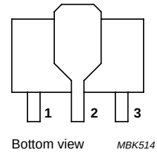
Fig.1 SOT89.
