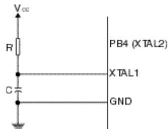
图 5 外部 RC 配置
