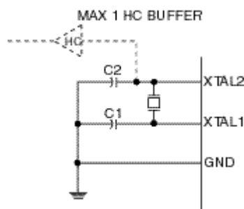
图 3 振荡器连接
