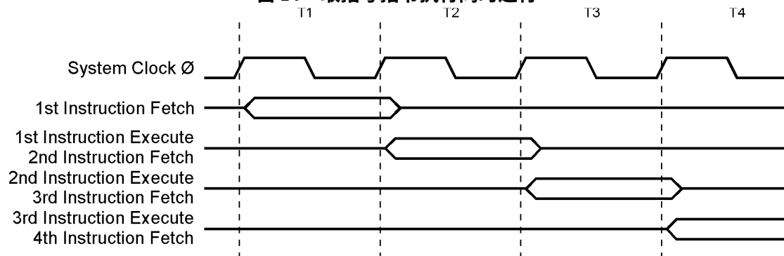
图 14 取指与指令执行同时进行
