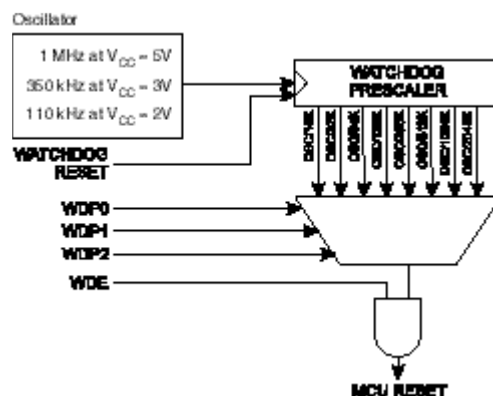
图 25 看门狗定时器
