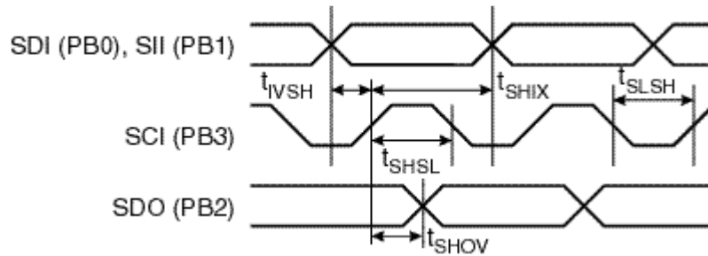
图 29 高压串行编程时序
