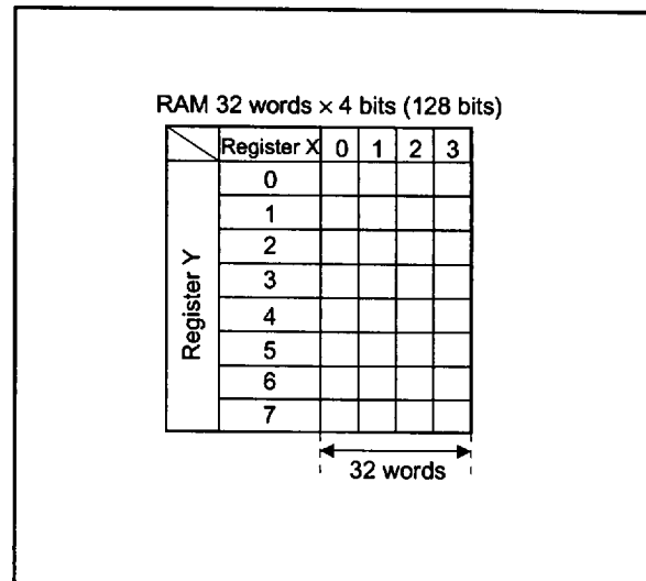
Fig. 11 RAM map
