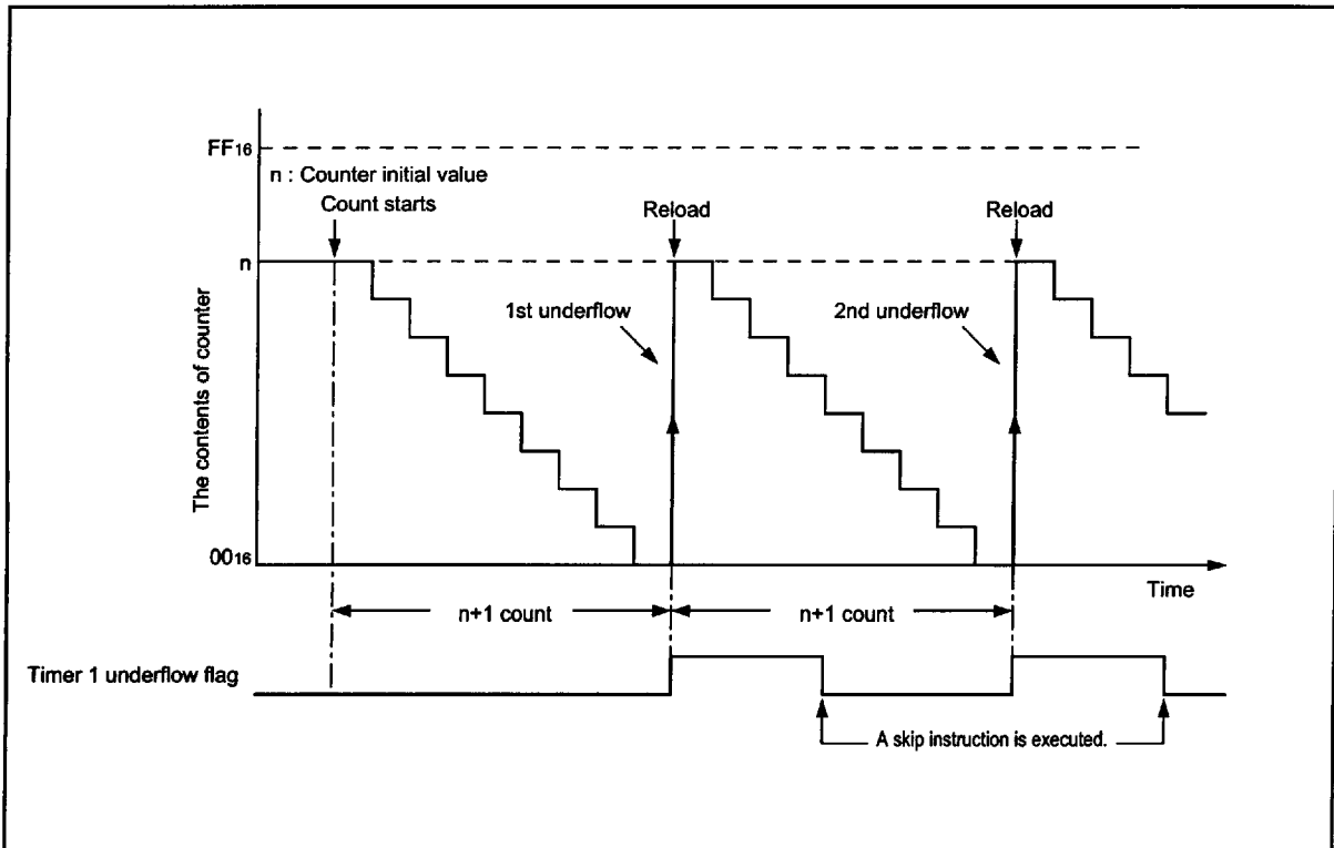
Fig. 12 Auto-reload function
