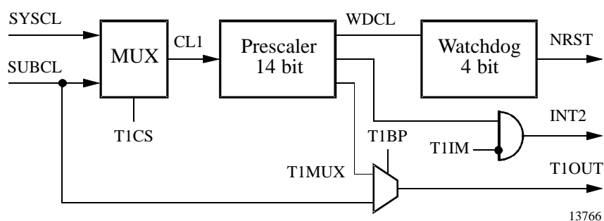
Figure 27. Timer 1 module
