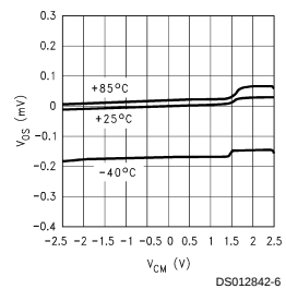
V_{OS} vs V_{CM} V_S = \pm 2.5\text{V}
