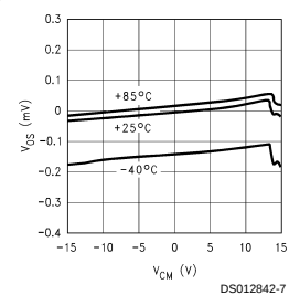
V_{OS} vs V_{CM} V_S = \pm 15\text{V}
