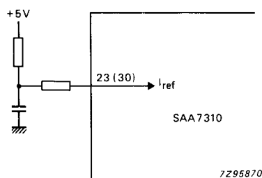
Fig. 13 I_{ref} circuit.
