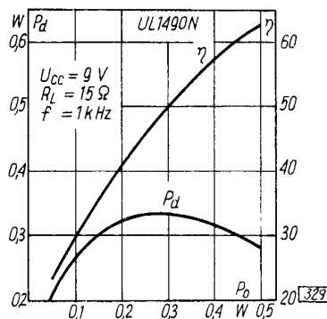
Moc strat i sprawności w funkcji mocy wyjściowej
