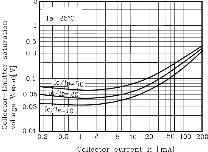
Fig. 5 V_{CE(sat)} - I_C
