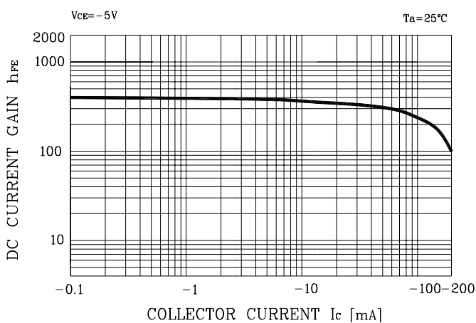
Fig. 1 h_{FE} - I_C
