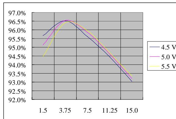
Vo=3.3 V
