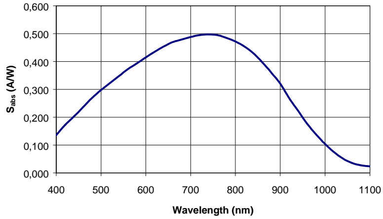
SSO - AD - serie Spectral Responsivity at M=100
