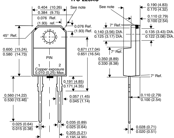
ITO-220AC
