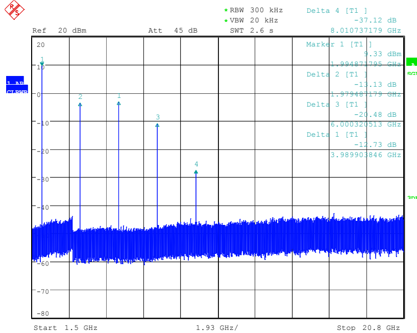
HARMONIC SUPPRESSION
