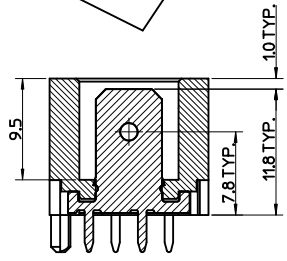
A-A Scale 3:1
