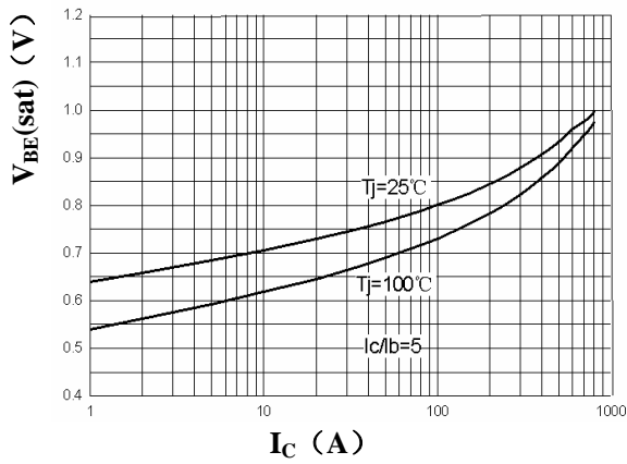
V_{BE(sat)} - I_C
