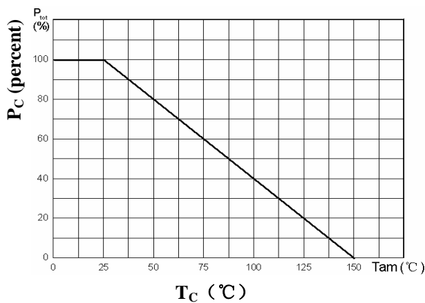
P_C - T_C
