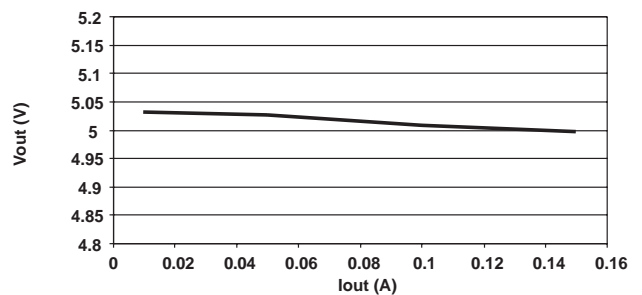
Vout Vs. Iout (PSM mode) Vin = 3V
