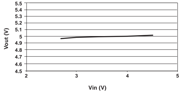
Vout Vs. Vin Iout = 500mA
