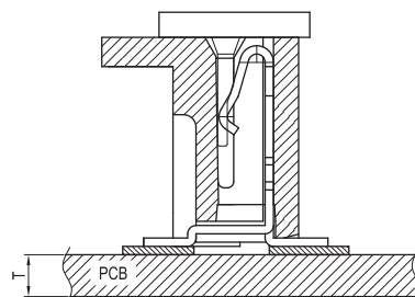
PCB ASS'Y
