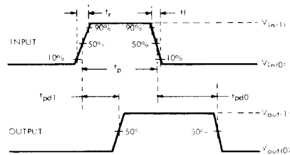
Dwg. No. A-7628C
