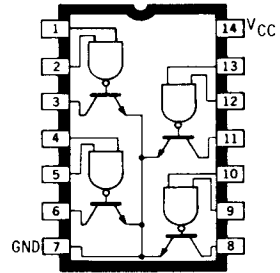
Dwg. No. A-7606
