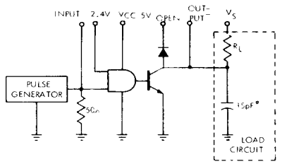
Dwg. No. A-7899C
