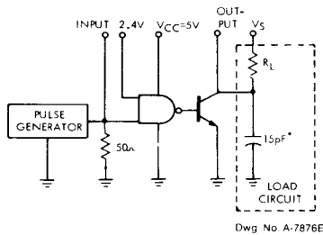
Dwg. No. A-7876E
