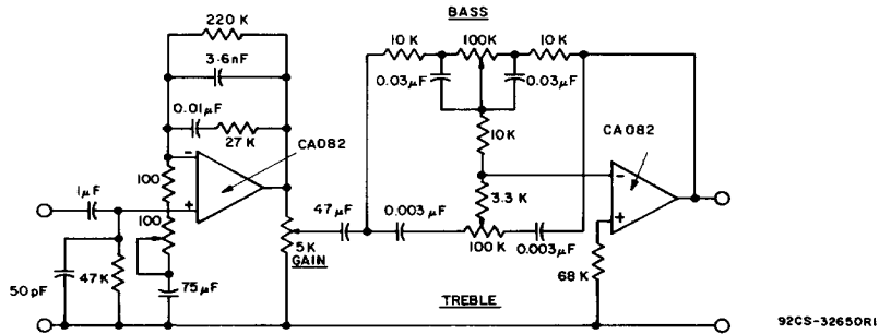
Fig. 19 - IC preamplifier.
