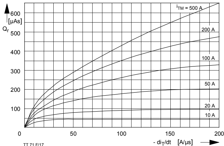
Bild / Fig. 17 Sperrverzögerungsladung Q_r = f(di/dt) t_{vj} = t_{vj \max} , v_R = 0,5 V_{RRM} , v_{RM} = 0,8 V_{RRM} Parameter: Durchlaßstrom I_{TM} / Recover charge Q_r = f(di/dt) t_{vj} = t_{vj \max} , v_R = 0,5 V_{RRM} , v_{RM} = 0,8 V_{RRM} Parameter: on-state current I_{TM}
