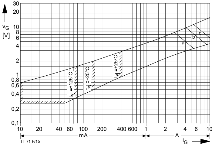
Bild / Fig. 15 Steuercharakteristik mit Zündbereichen / Gate characteristic with triggering areas, v_G = f(i_G) , v_D = 6 V
