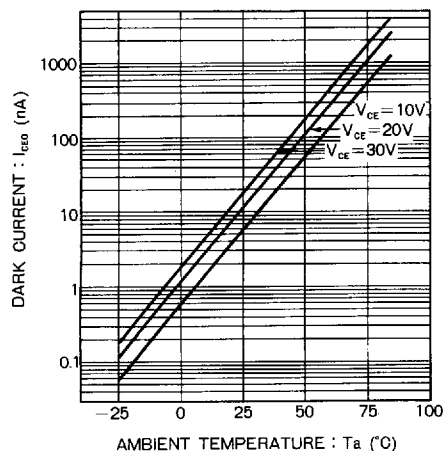
Fig.1 暗電流-周囲温度特性
