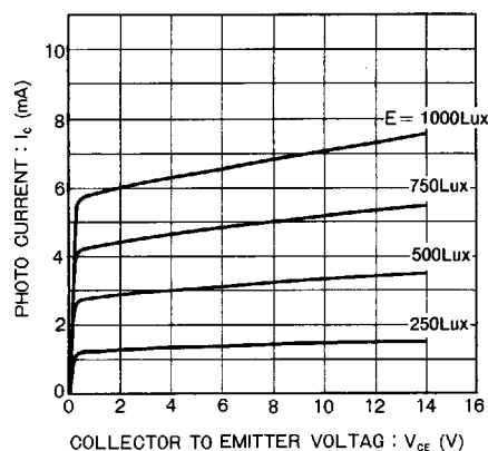
Fig.4 光電流-コレクタ・エミッタ間電圧特性
