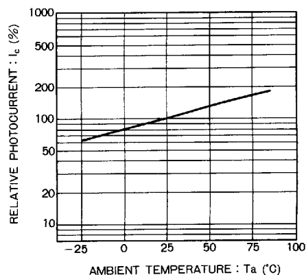
Fig.2 光電流-周囲温度特性
