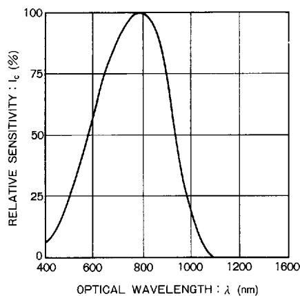
Fig.5 分光感度特性
