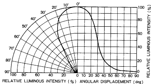
Fig.6 指向特性
