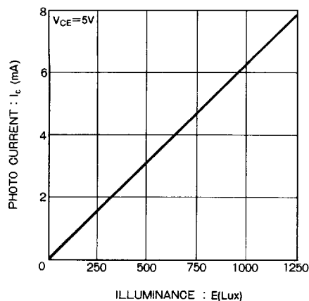
Fig.3 光電流-放射照度特性
