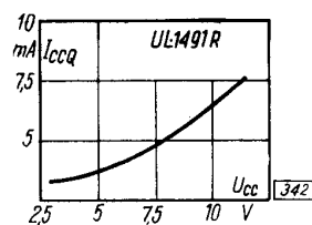
Prąd spoczynkowy zasilania w funkcji napięcia zasilania
