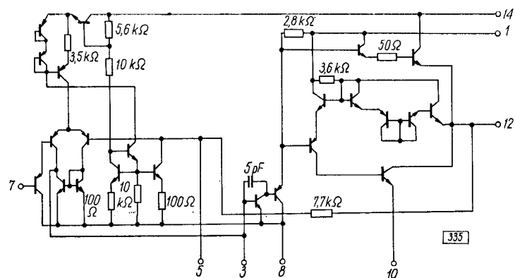
Schemat elektryczny
