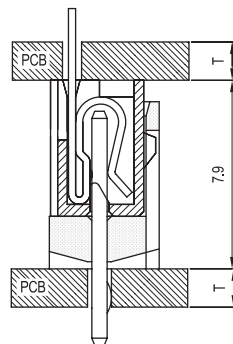
PCB ASS'Y
