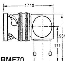
3-lug ADRMF70 2-lug ADRMF70TL Threaded ADRMF370 4-lug ADRMF70FL
