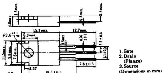
(JEDEC TO-220AB)
