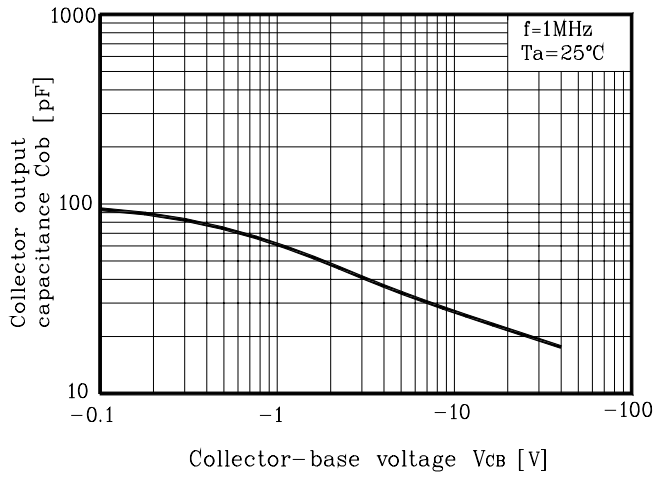
Fig. 7 C_{ob} - V_{CB}
