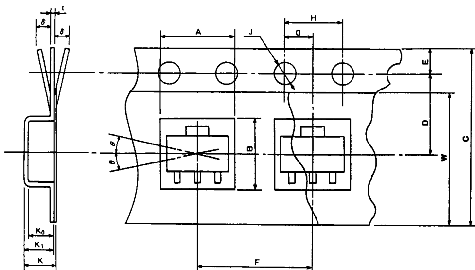
Taping dimensions
