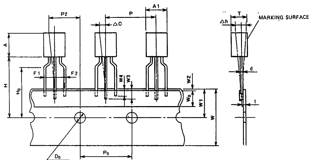
Taping dimensions
