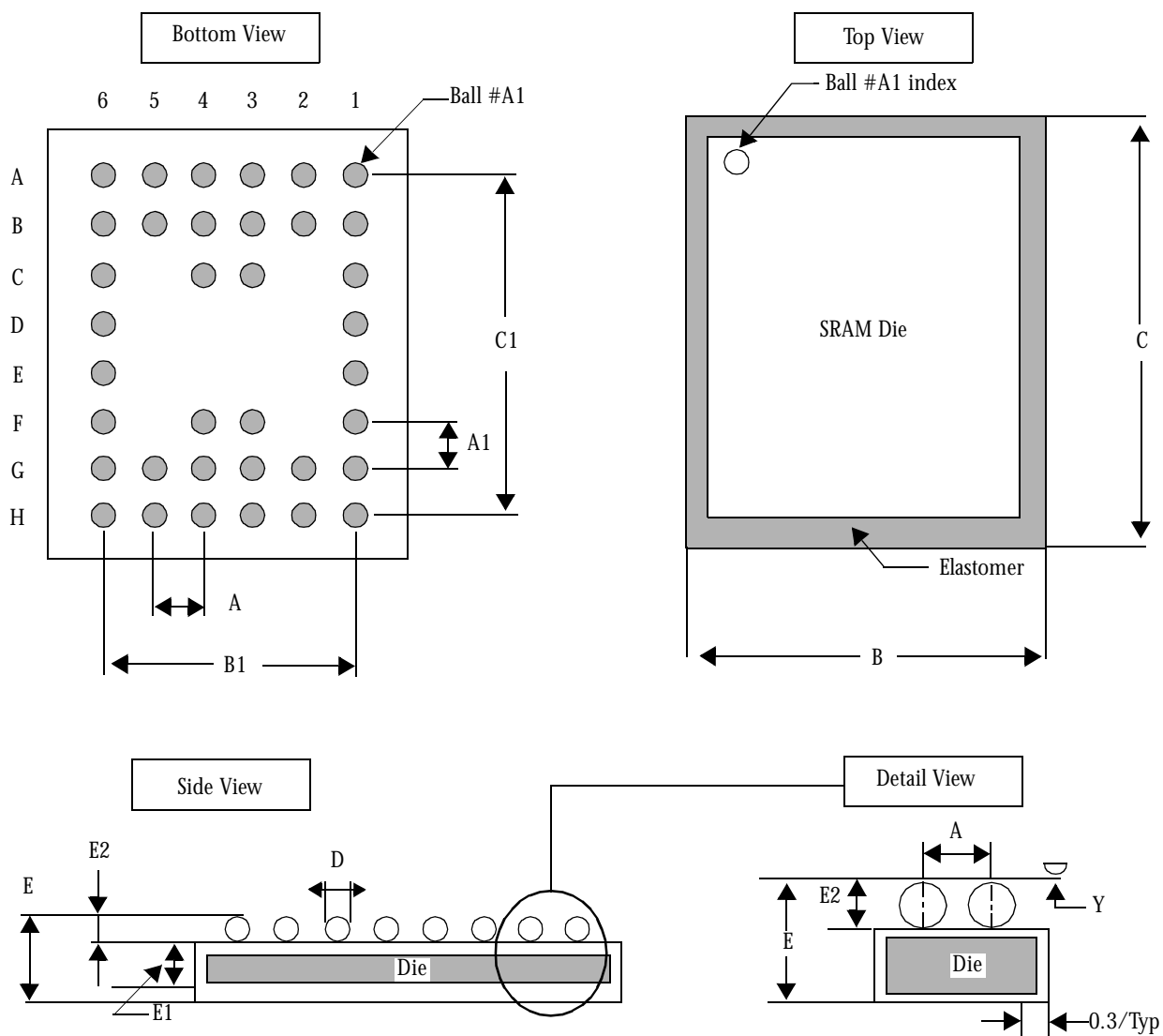
36(48)-ball FBGA
