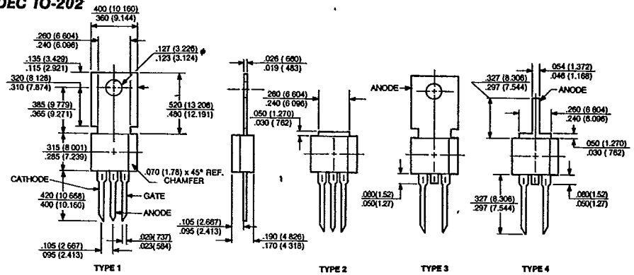
JEDEC TO-202
