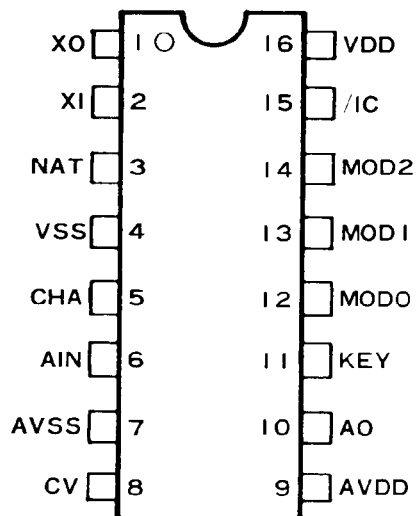
<16DIP Top View>
