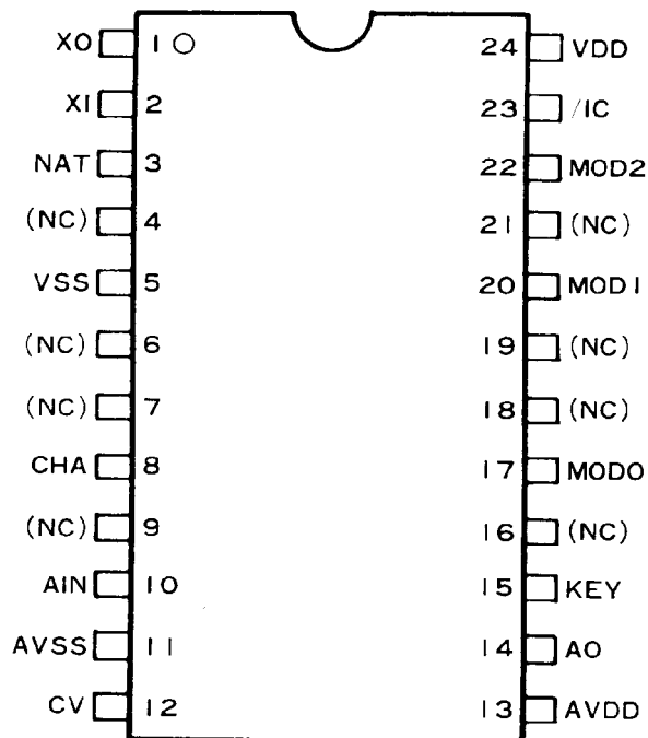
<24SOP Top View>
