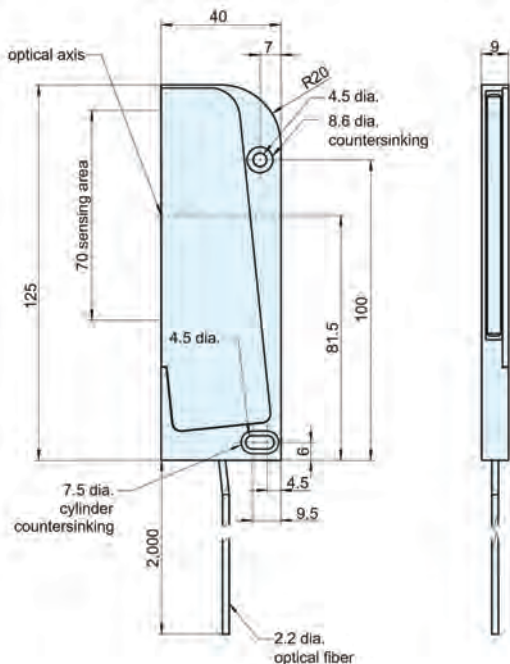
E32-T16P E32-T16PR
