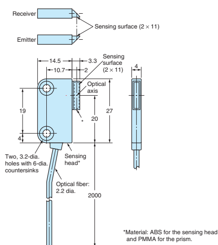
E32-T16J E32-T16JR
