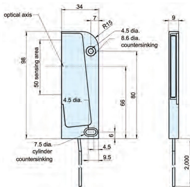
E32-T16
