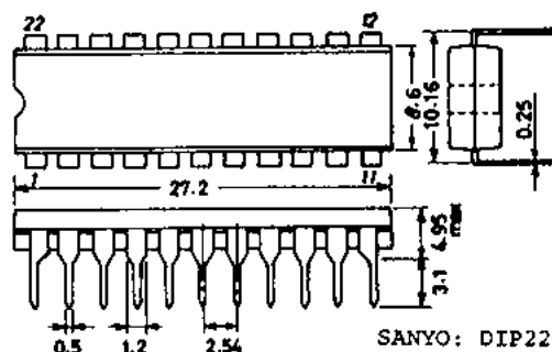
外形図 3010A-D22IC (unit: mm)
