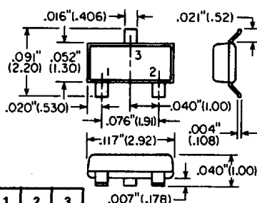
SOT-23
