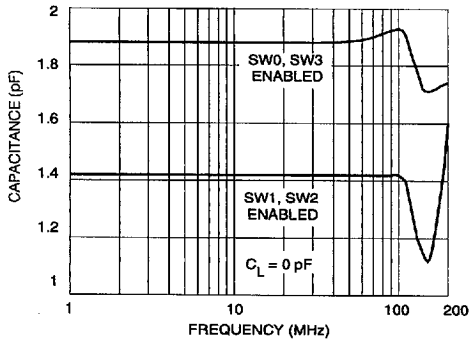
Fig. 3 Input Capacitance
