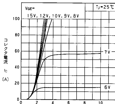
出力特性(標準値) Typical Output Characteristics
