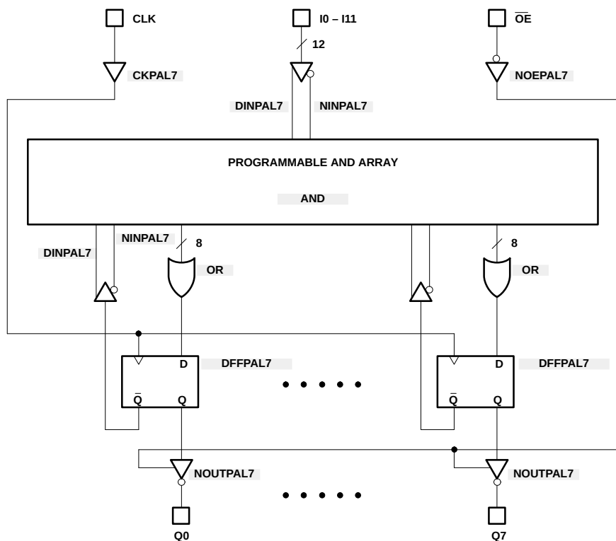
PLUS20R8
