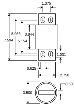
Fig. 2: 900-1000 Amp Range
