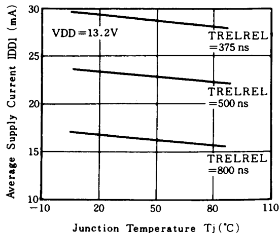
IDD1 vs. Tj
