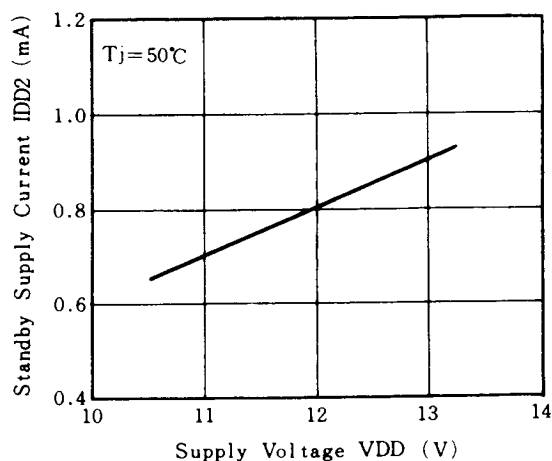
IDD2 (STANDBY) vs. VDD
