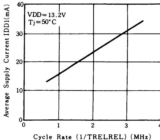
IDD1 vs. CYCLE RATE
