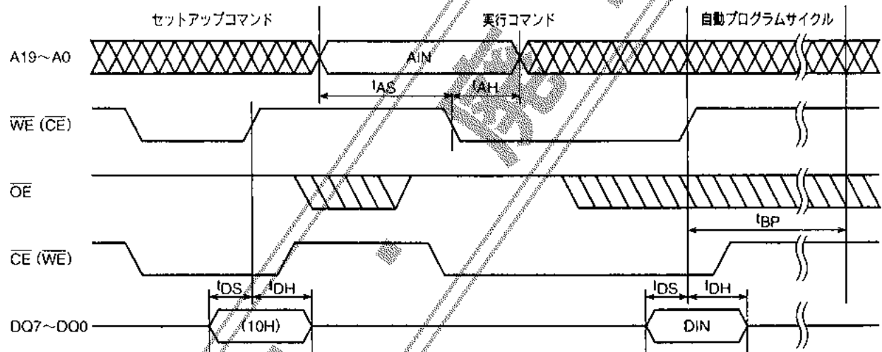
図7: バイトプログラム
