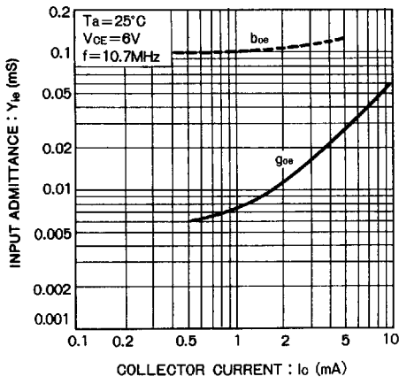
Fig.17 入力アドミタンスーコレクタ電流特性
